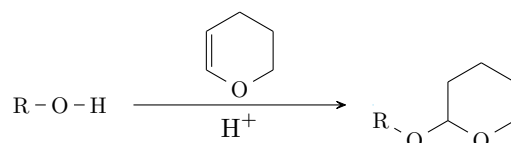
FIGURE 10.6 – Protection d'un alcool par le DHP
